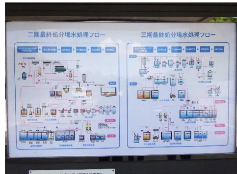
水処理施設処理フロー
